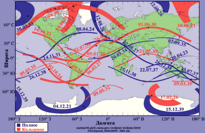
Пути полных и кольцевых солнечных затмений в 2021-2040 гг.
